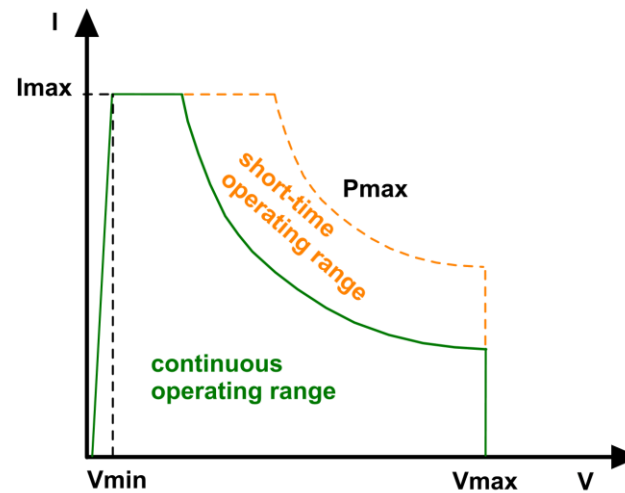
Abbildung 2.14: Betriebsbereich Figure 2.14: Operating range
