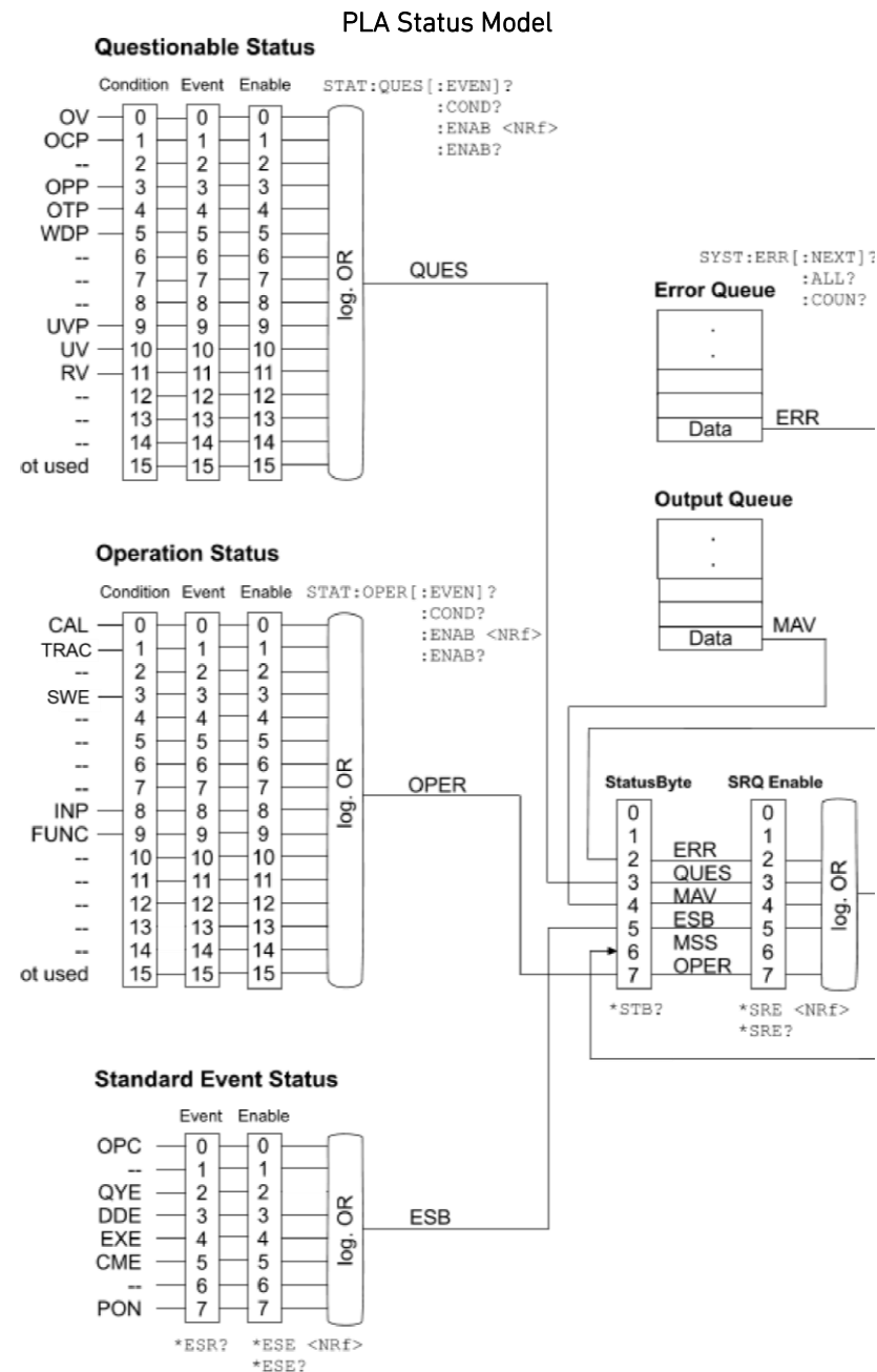
Abbildung 5.2: PLA Statusmodell
