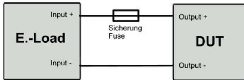
Abbildung 2.15 Verpolschutz durch Sicherung oder Diode Figure 2.15: Reverse voltage protection by fuse or diode
