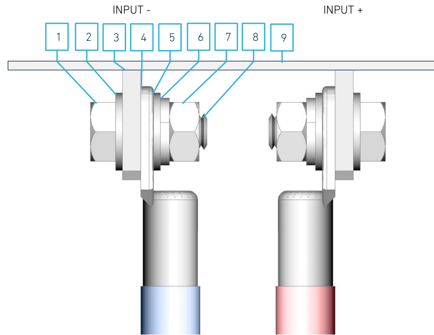
Abbildung 2.13: Anordnung der Schrauben und Scheiben an der Stromschiene Figure 2.13: Sequence of screws and washers at output terminal
