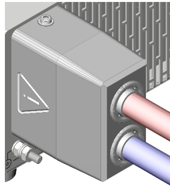
Abbildung 2.12: Abdeckhaube mit durchgeführten Lastleitungen Figure 2.12: Cover with load lines fed through
