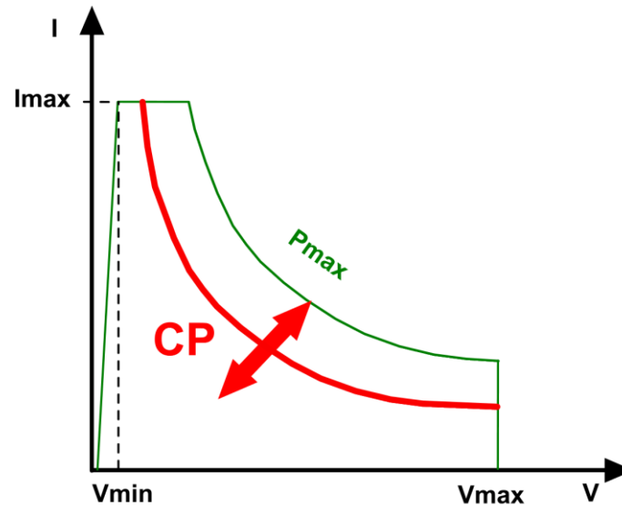
Abbildung 3.2: Konstantleistungsbetrieb (CP)
