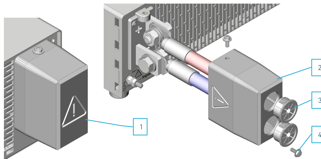
Abbildung 2.11: Sicherheitsabdeckung für unbenutzte (l) und angeschlossene (r) Lastleitungen Figure 2.11: Safety cover for unused (l) and for connected (r) input terminals
