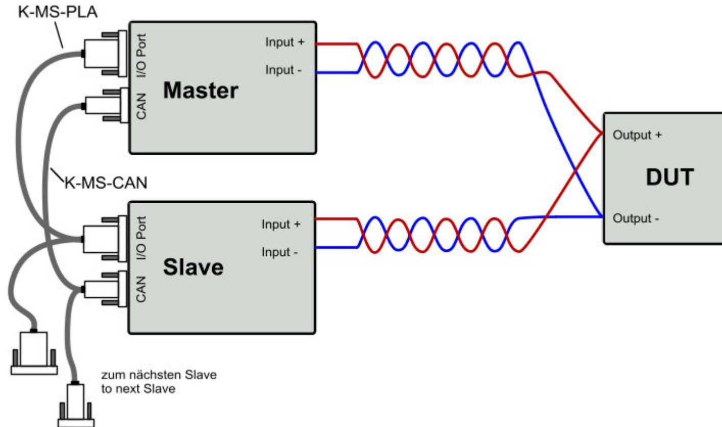
Abbildung 3.8: Verschaltung im Master-Slave-Mode Figure 3.8: Wiring in Master-Slave mode
