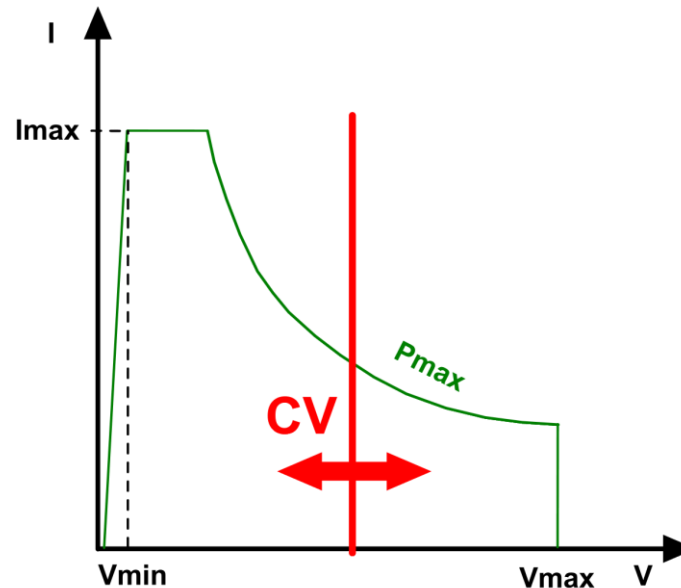
Abbildung 3.4: Konstantspannungsbetrieb (CV)
