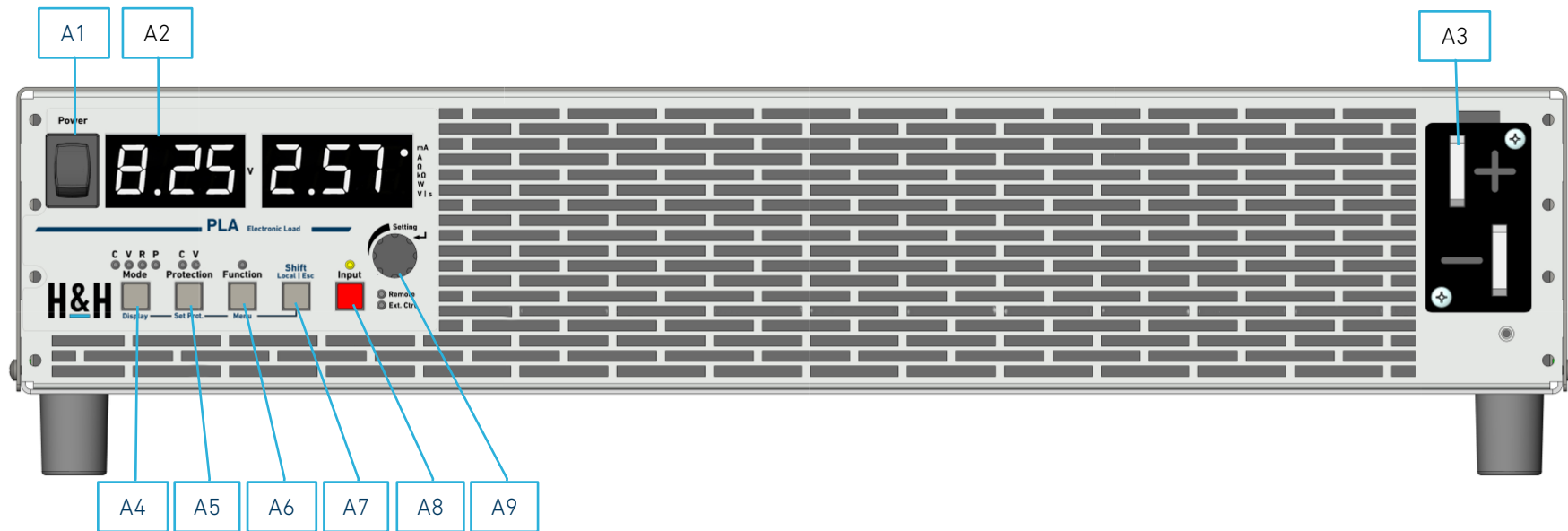
Abbildung 2.3: Bedienelemente PLA8xx/PLA12xx
