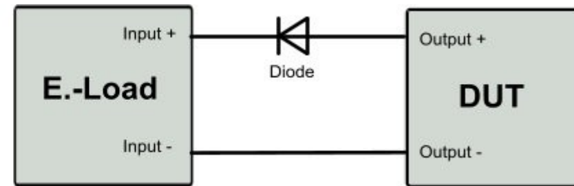
Abbildung 2.15 Verpolschutz durch Sicherung oder Diode Figure 2.15: Reverse voltage protection by fuse or diode
